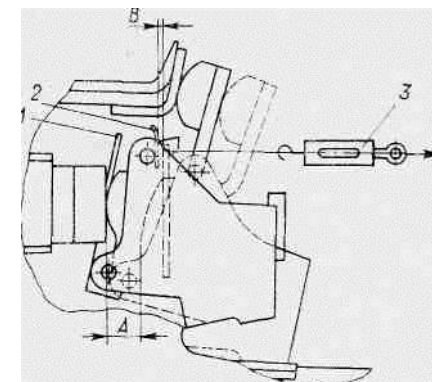
Рис. 7. Параметры контактной системы главных контактов: 1 — бумажная полоска при измерении R_{нач} ; 2 — бумажная полоска при измерении R_{кон} ; 3 — динамометр; L — раствор; B — зазор, контролирующий провал
