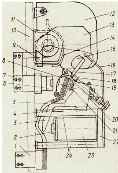
Рис. 2. Контактор:
